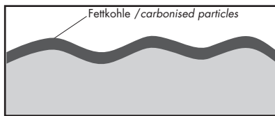
Fettkohle / carbonised particles Fettkohle-Haftung bei oberflächenvergütetem Edelstahl. Adhesion of carbonised particles on a treated surface
