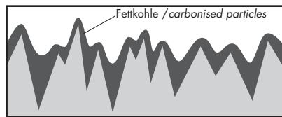
Fettkohle / carbonised particles Fettkohle-Haftung bei unbehauelter Edelstahloberfläche. Adhesion of carbonised particles on a normal surface
